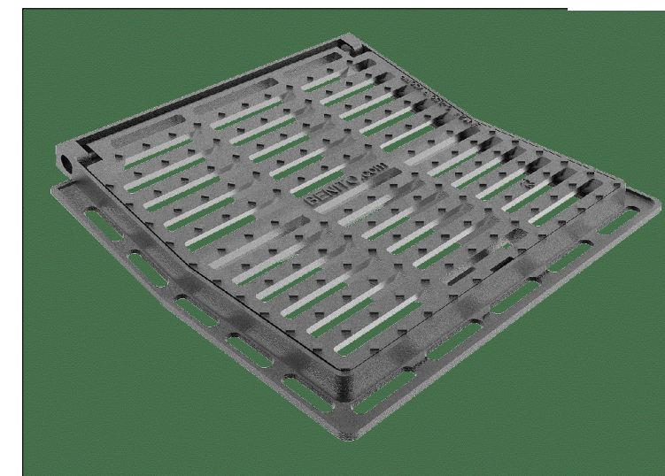
Reixa de recollida d'aigües pluvials Model Cóncava 60*60.-cm de "Benito Urban" o similar
